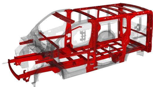
Structure renforcée
