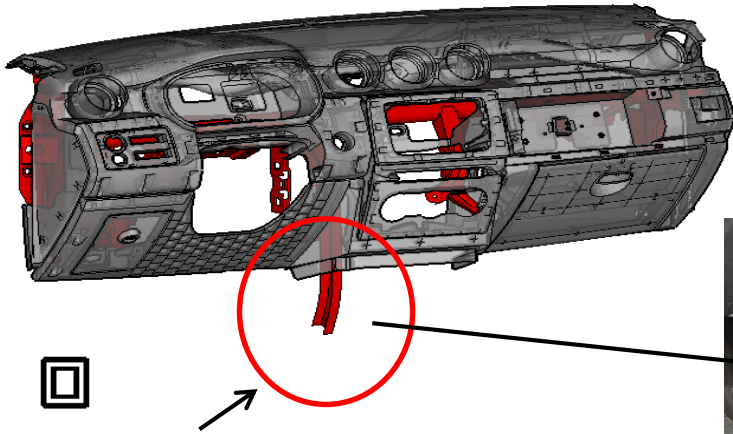
Présence de renfort latéral sous la console centrale , côté conducteur
